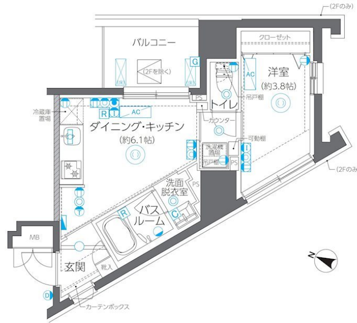
【間取り図】
