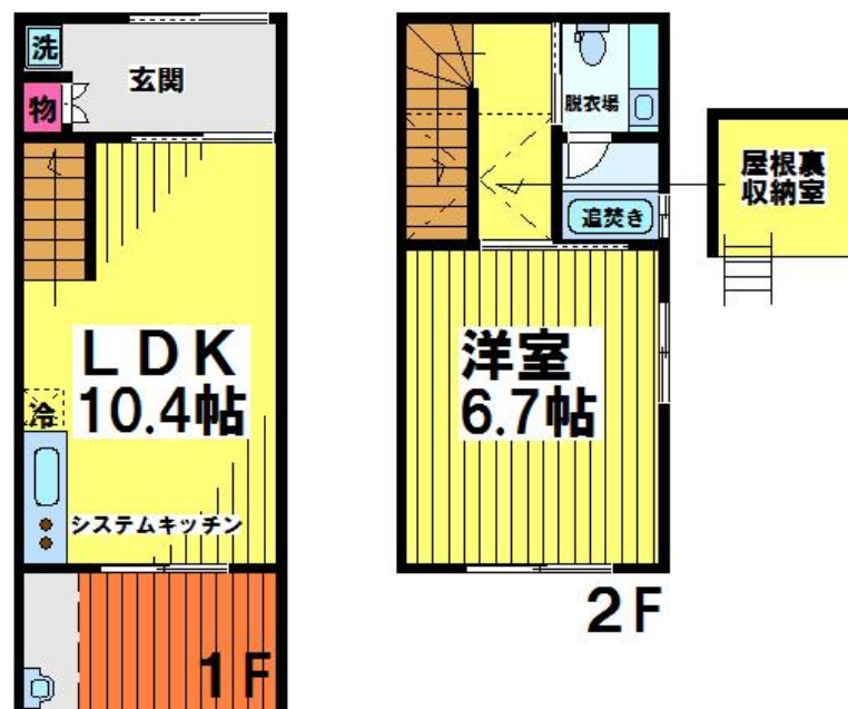
【問取り図】
