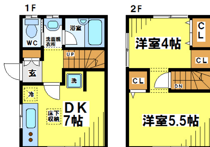
【間取り図】
