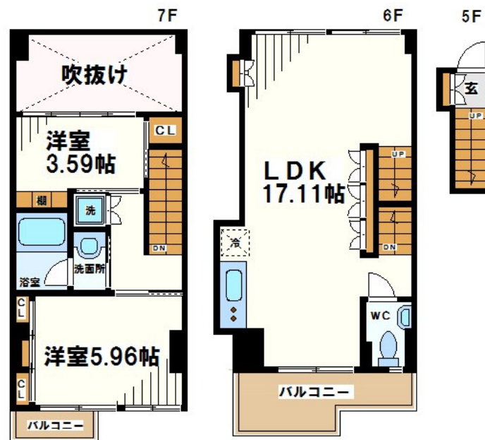
【間取り図】
